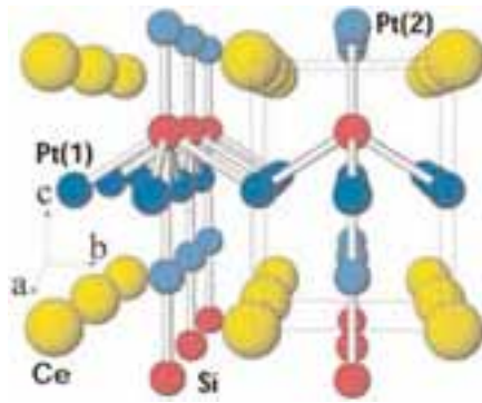
Abb. 1: Kristallstruktur von \text{CePt}_3\text{Si} . Die Struktur ist tetragonal, zeigt aber in Richtung der polaren c-Achse kein symmetrisches Verhalten (= Fehlen eines Inversionszentrums)
