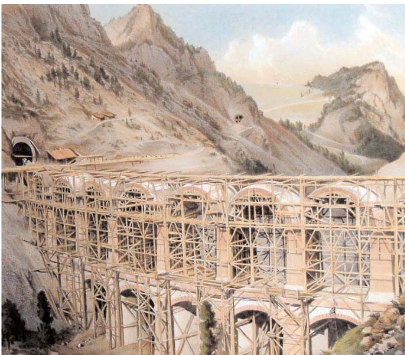
Blick auf die Eisenbahntrasse unter dem Adlitzgraben – die Gewölbe der oberen Bogenreihe sind bereits fertiggestellt, es fehlt nur der Aufbau zum Gleisbett
