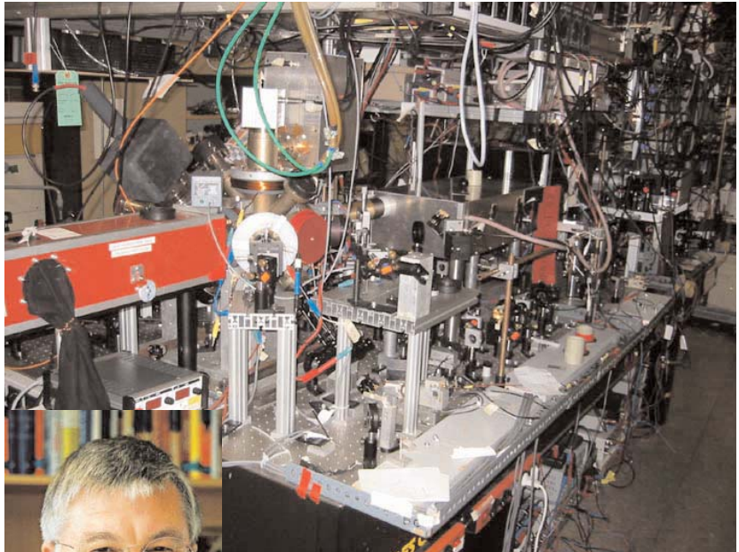
Versuchsanordnung in der Universität Innsbruck
