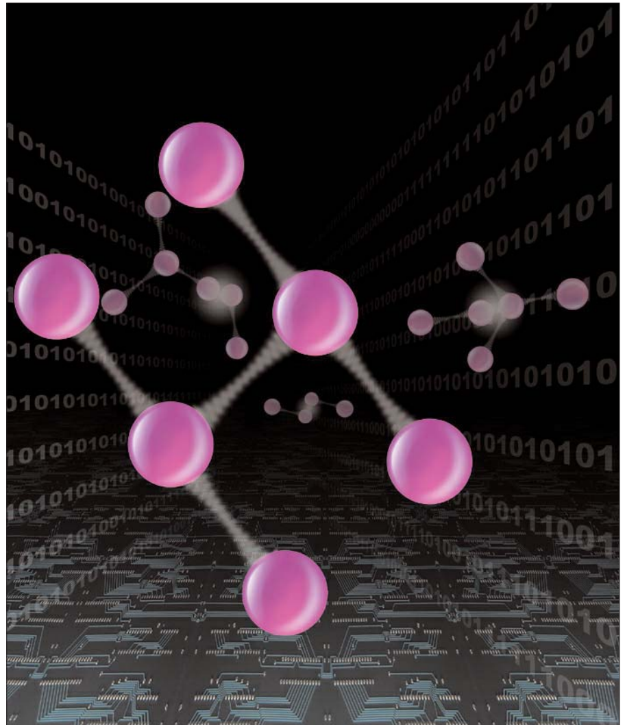
Illustration des verschränkten Sechsfotonenzustands
