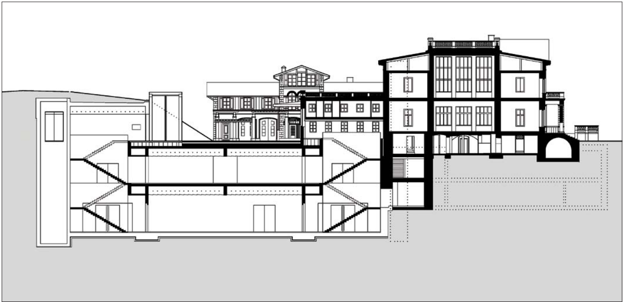
Schnittzeichnung durch die Villa Wesendonck und den Erweiterungsbau. Es wird deutlich, wie ein Teil der neuen Räume unter die Villa »geschoben« wurden. Sichtbar ist nur der »Smaragd«, der Eingang.
