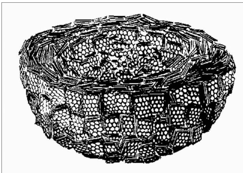
Schnittzeichnung eines Rußprimärpartikels
