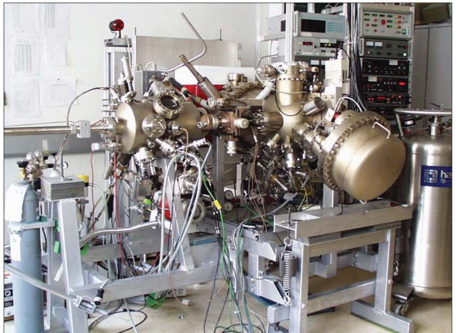
Ein Rastertunnelmikroskop
