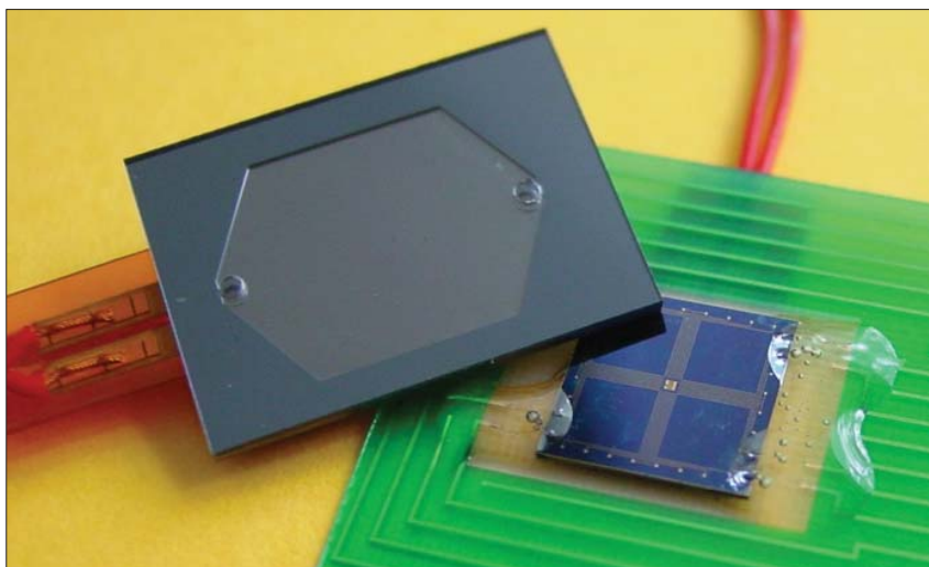
PCR-Kammer und Goldelektroden-Chip zur DNA Detektierung
