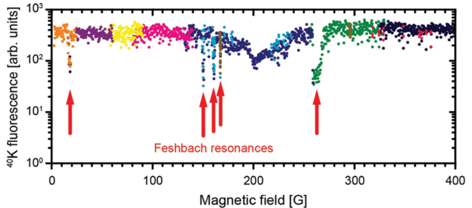
Auschnitt der experimentellen Daten der Feshbach Resonanzen. Nur für ganz bestimmte Magnetfelder ist die Wechselwirkung der Atome so groß, daß hohe Verluste auftreten.
