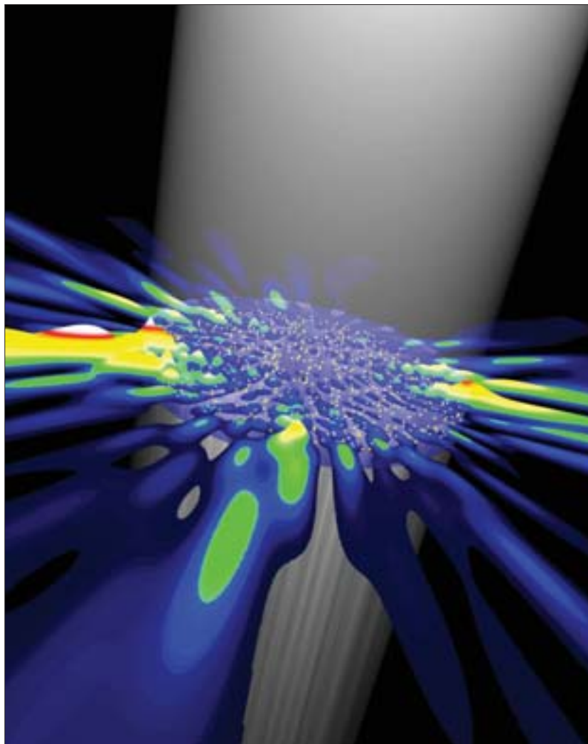
Ein Zufallslaser wird von oben bestrahlt und sendet in zufällige Richtung Laserlicht aus – By Robert Tandy & Science Magazine
