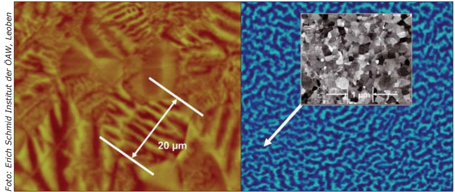
Stahl vor seiner Verformung (li.) und danach (re.) im Magnetkraftmikroskop. Das Raster-Elektronenmikroskop macht die einzelnen Nanokristalle sichtbar
