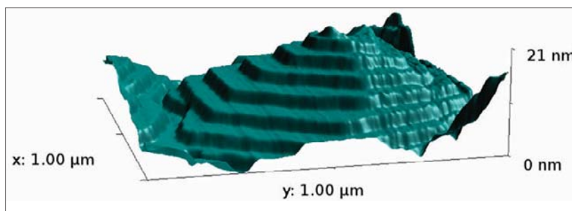
Rasterkraftmikroskopieaufnahme eines terrassierten Hügels aus aufrecht stehenden organischen Molekülen. Die Terrassenhöhe entspricht der Moleküllänge.
