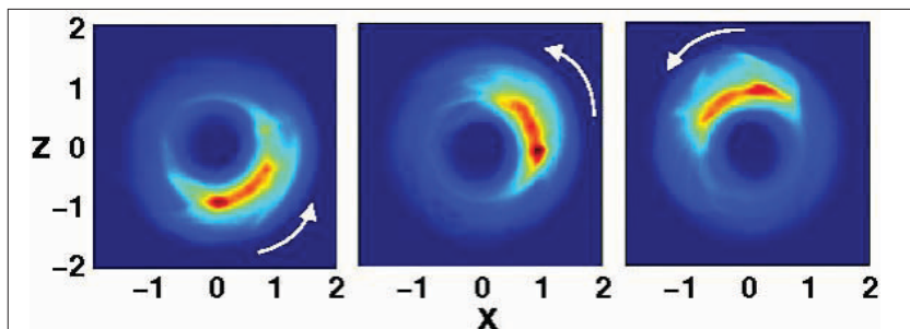
Drei Momentaufnahmen zu verschiedenen Zeiten des Wellenpakets, das den Kern eines Kaliumatoms auf einer Umlaufbahn umkreist. Sie zeigen die Erzeugung eines Bohratoms.
