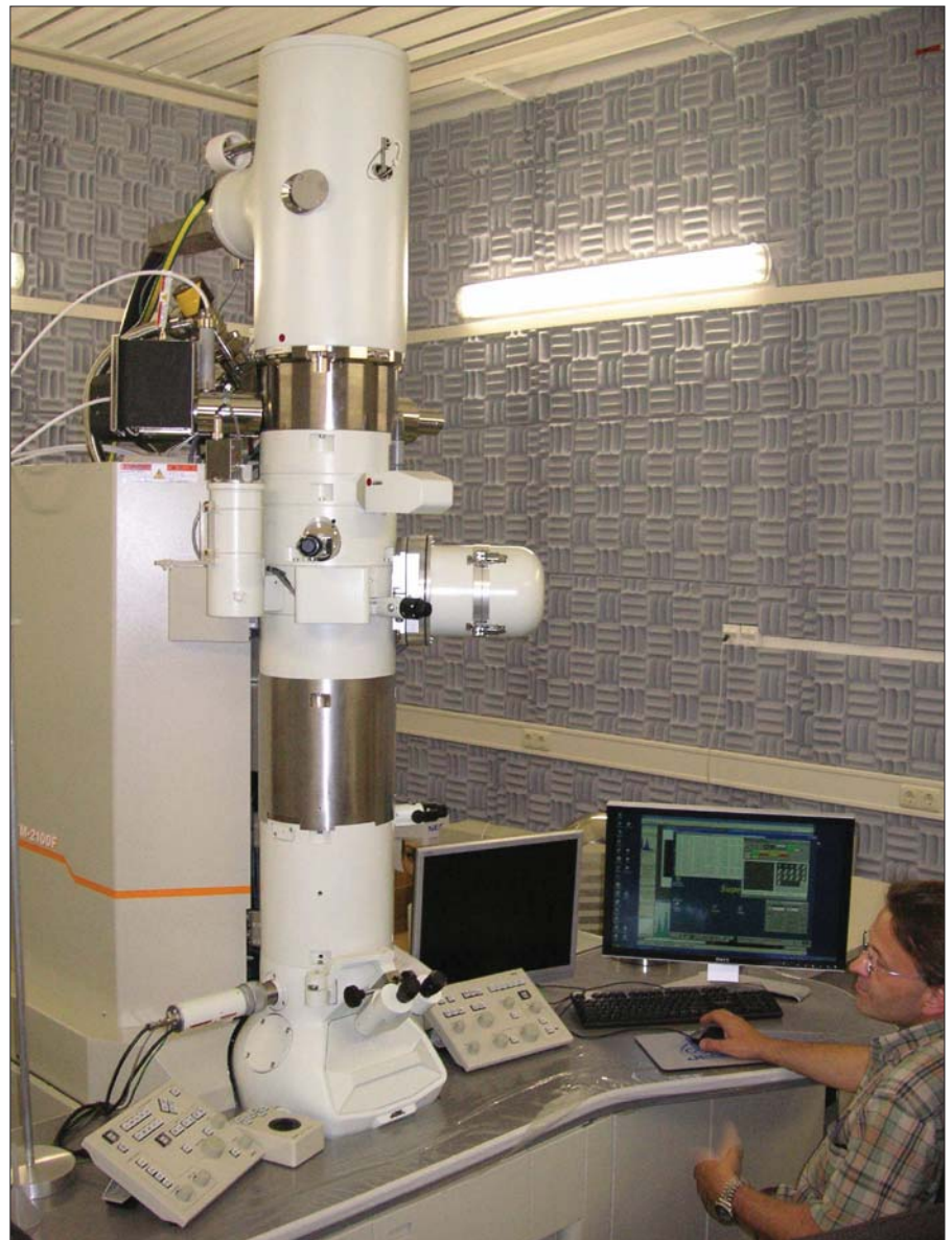
Das JEM JEOL 2100F ist das derzeit einzige mit Cs-Korrektor ausgestattete Transmissionselektronenmikroskop in Österreich
