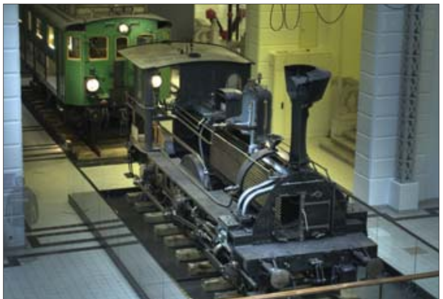
Die 1883 gebaute »Schnittlok« veranschaulicht die Funktionsweise einer Dampflokok
