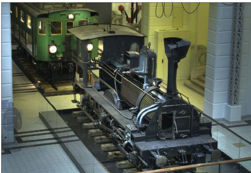
Die 1883 gebaute »Schnittlok« veranschaulicht die Funktionsweise einer Dampflokom
