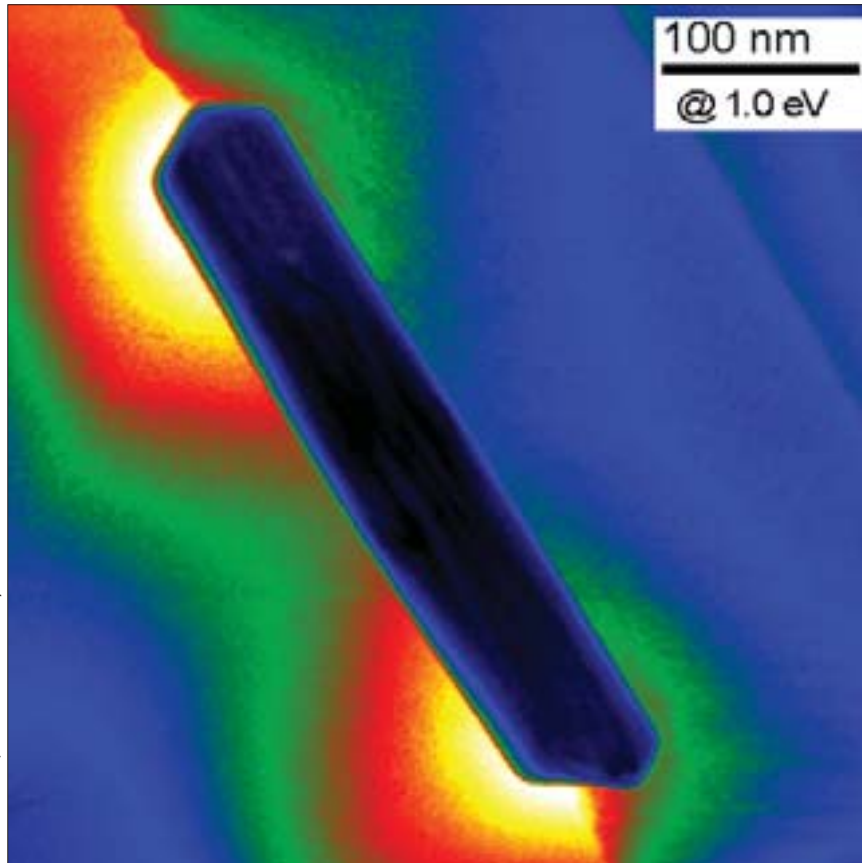
Oberflächenplasmon auf einem Goldteilchen im Nanometer-Bereich
