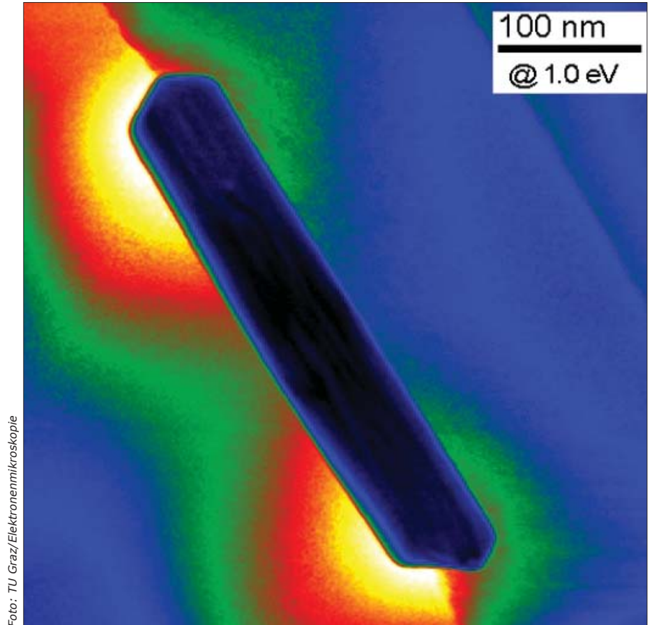
Oberflächenplasmon auf einem Goldteilchen im Nanometer-Bereich
