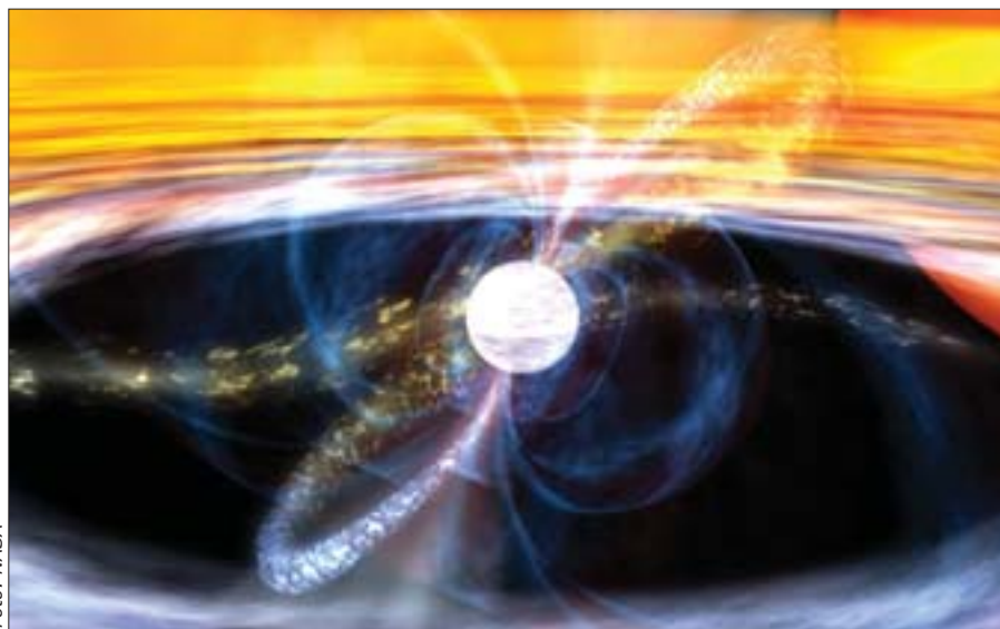
Ein Millisekundenpulsar mit der Nachbarsonne im Hintergrund
