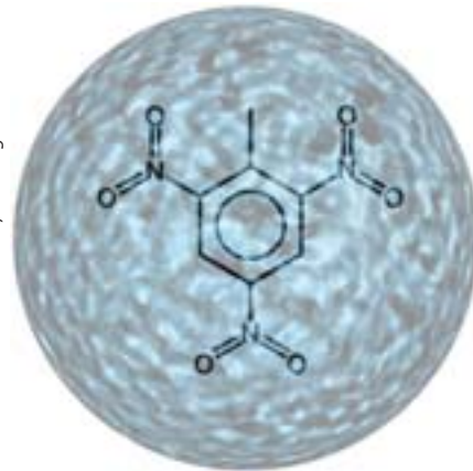
Um den Zerfall von TNT zu studieren, hat Paul Scheier mit seinem Team die Explosion des Sprengstoffs in ultrakalten Heliumtröpfchen quasi eingefroren.
