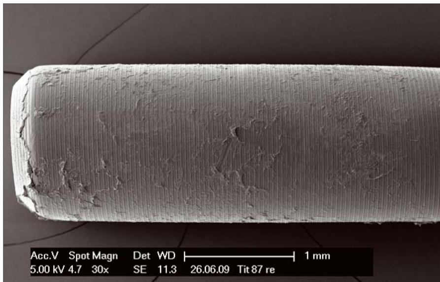
Implantatstift aus Titanlegierung nach 1-monatiger Implantation: erste Knochen-gewebeteile haben sich gebildet.
