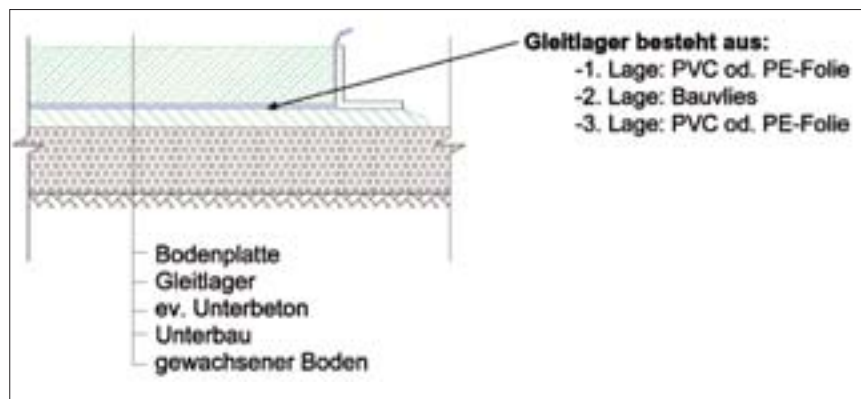
Abb. 2 Schematischer Aufbau der neuartigen Gleitlagerung
