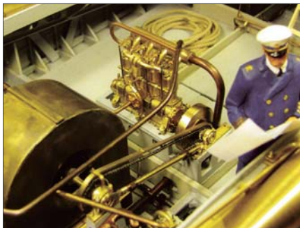
Detail aus dem Modell von G. Schuster
