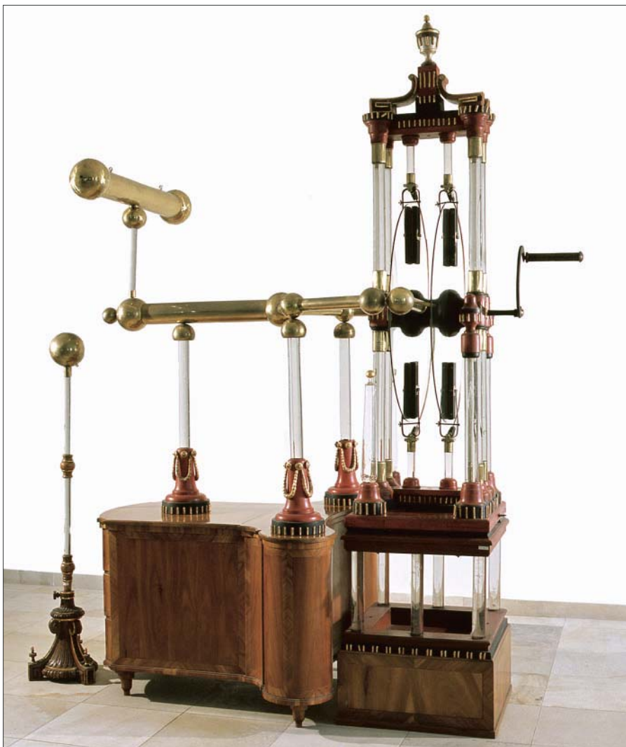
Scheibenelektrisiermaschine, angefertigt von Johann Jechl nach Anleitung des Jesuitenpaters Franz Xaver Racher, Linz-Krummau 1794; Oö. Landesmuseen
