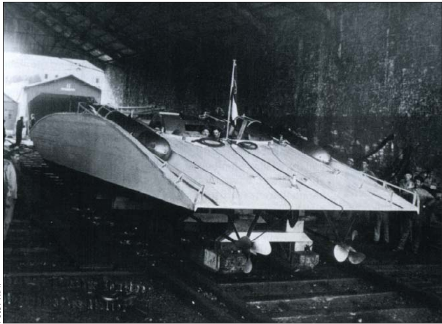
Heckansicht des Versuchs-Gleitbootes auf der Helling in Pola; man beachte den scharfen Hecksteven, die Propeller und das Heckruder.
