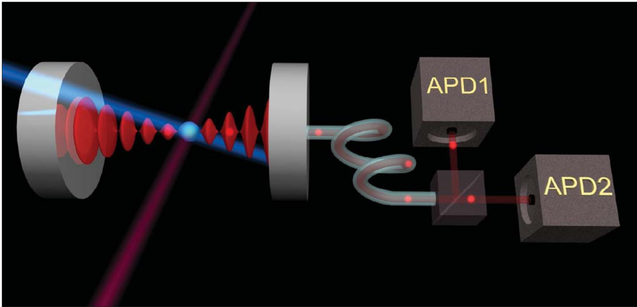
Abbildung des Einzelatomlasers. Ein einzelnes gefangenes Ion (blaue Kugel) ist umgeben von einem optischen Resonator und wird von externen Lasern angeregt, wobei es Laserlicht in den Resonator emittiert. Das Licht verlässt den Resonator durch einen der beiden Spiegel und wird über eine optische Faser zu den Detektoren geführt. Foto: Universität Innsbruck / Schmidt
