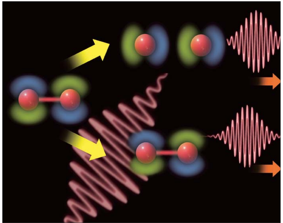
Ein Molekül (links) wird in einen Überlagerungszustand aus "zerbrochen" (oben) und "ganz" (unten) versetzt. Ein Laserpuls kann das Molekül (bzw. die Atome) dazu anregen, ihrerseits Licht auszusenden (rechts).
