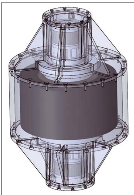
Skizze des Schwungrades mit Karbon-Mantel
