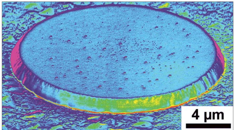
Rasterelektronen-Mikroskopieaufnahme eines Infrarot-Mikrodisk-Lasers
