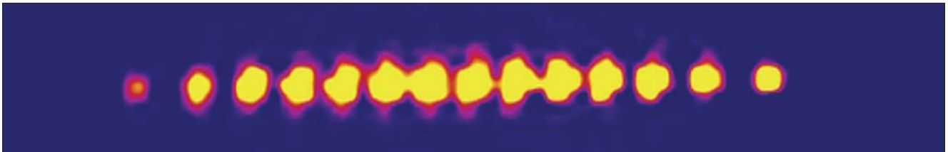
14 Quantenbits wurden von Innsbrucker Quantenphysikern in einer Ionenfalle miteinander verschränkt.
