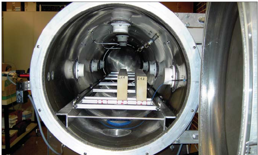
Das Holz wird in eine Imprägnierlösung mit siliziumoxidischen Solen getaucht und in einer Mikrowelle getrocknet.
