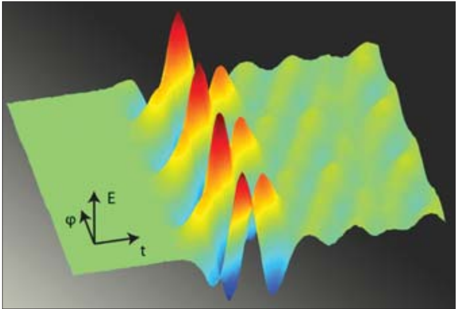
Gepulste Terahertz-Wellen, erzeugt mit maßgeschneiderten Ultrakurzlichtpulsen
