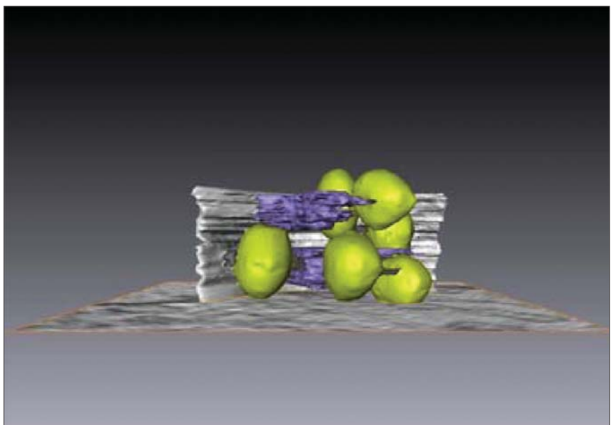
Vorher (oben)/nachher: Aufnahme einer Synapse zwischen zwei Nervenzellen; unten: Aufnahme mittels Elektronentomographie – aus Kippserien erstelltes 3D-Modell einer Synapse mit den Vesikeln gelb, dem Halteapparat violett und der Zellmembran weiß.
