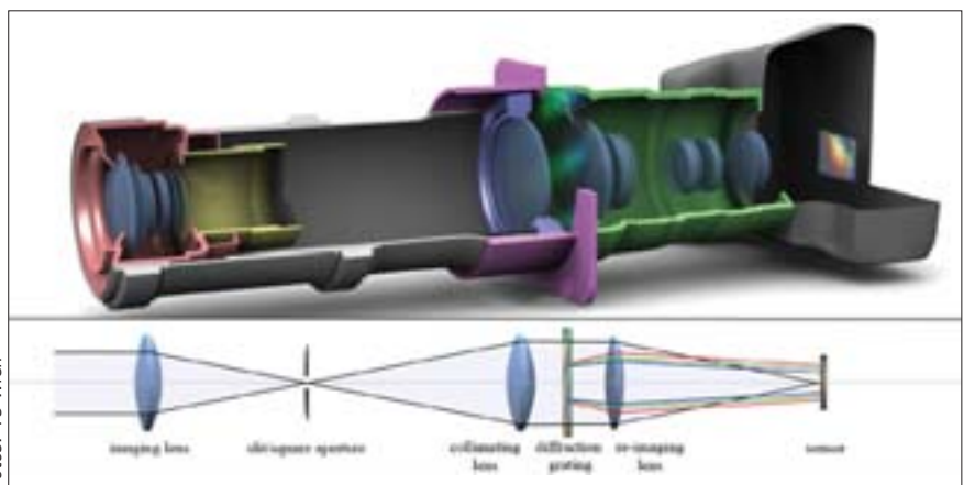
Schnitt durch die Spektral-Kamera, mit Strahlengang
