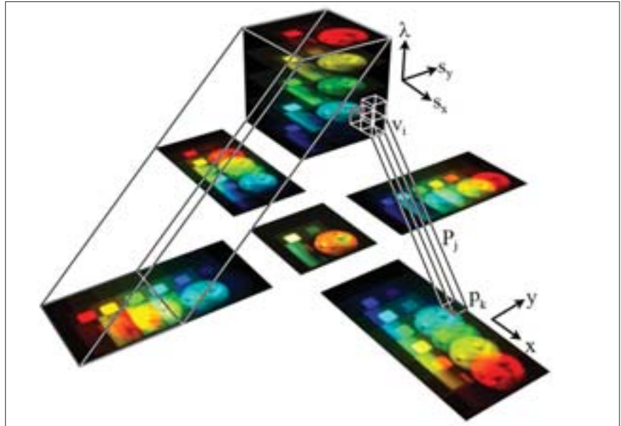
Gesucht wird eine dreidimensionale Datenstruktur: Zu jedem Punkt im Bild gibt es eine ganze zusätzliche Achse mit der spektralen Farb-Information. Am Sensor kommen Projektionen dieser Datenstruktur an – aus ihnen kann rechnerisch auf die eigentliche dreidimensionale Datenstruktur zurückgerechnet werden.
