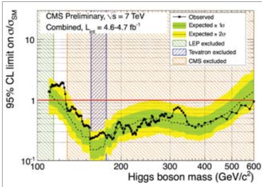
Obere Grenze für die Produktionsrate von Higgs-Bosonen im Vergleich zur Vorhersage des Standardmodells. Die gemessenen Daten schließen Werte über der schwarzen Linie mit einem Konfidenzniveau von 95 % aus. Die schraffierten Flächen entsprechen den existierenden Massengrenzen von LEP und dem Tevatron und dem neuen CMS-Resultat. Die gestrichelte Linie und die farbigen Bänder um diese Linie entsprechen der erwarteten Kurve und der Schwankungsbreite für hypothetische CMS-Experimente ohne Produktion von Higgs-Bosonen.
