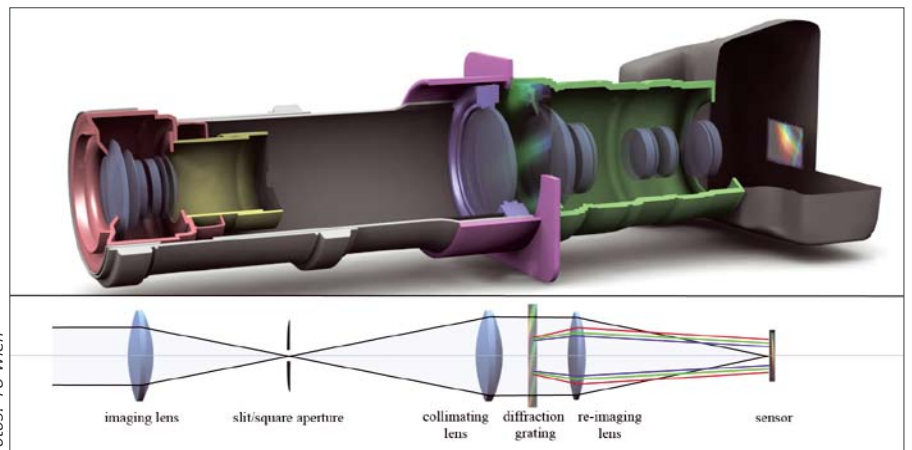
Schnitt durch die Spektral-Kamera, mit Strahlengang
