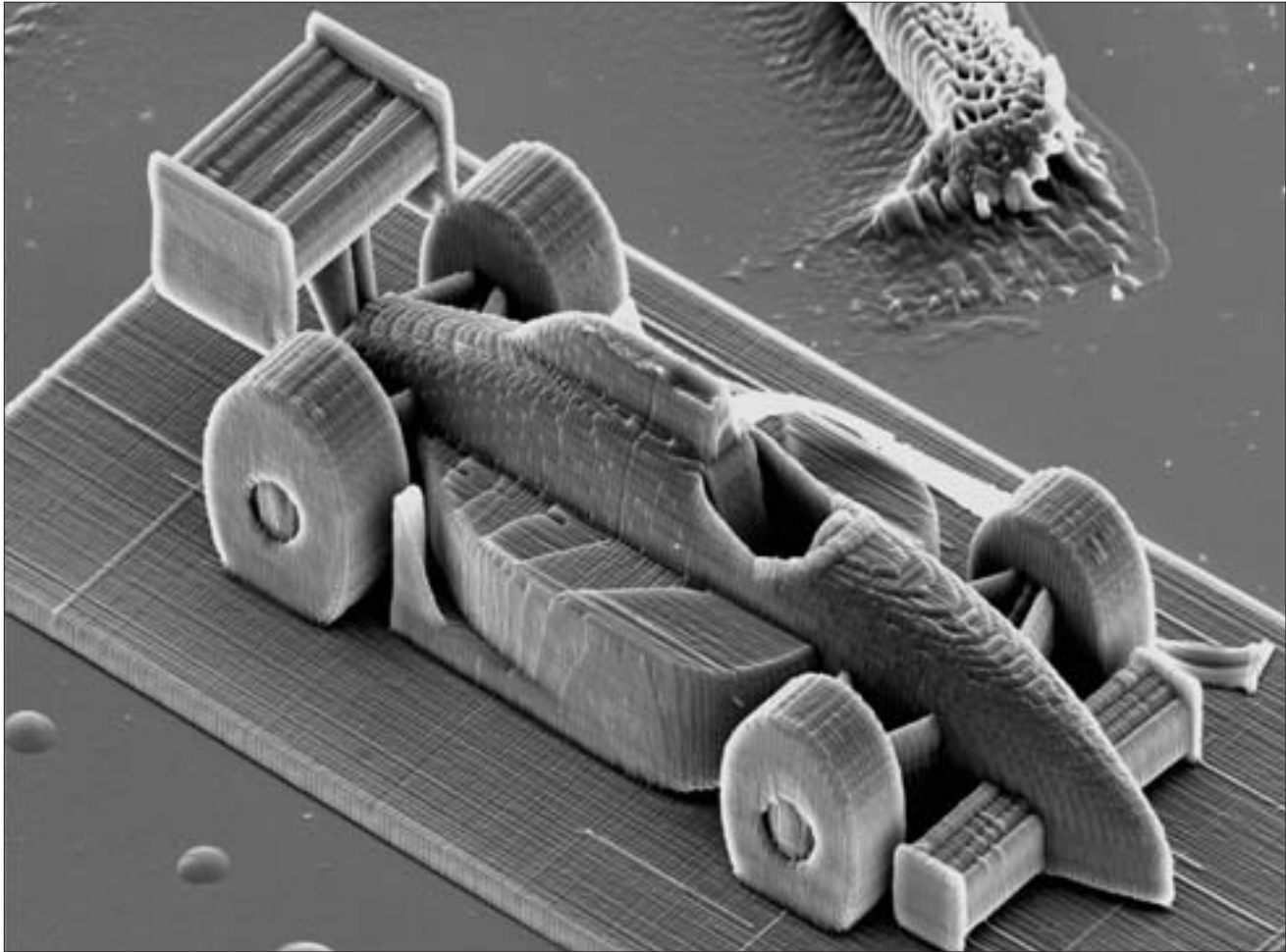
Rennauto mit ca. 285 µm Länge, gedruckt an der TU Wien. Der Brennpunkt des Laserstrahls wird mit beweglichen Spiegeln durch das Harz gelenkt und hinterläßt dort eine ausgehärtete Polymer-Linie mit einem Durchmesser von weniger als einem Zehntausendstel Millimeter (100 µm).
