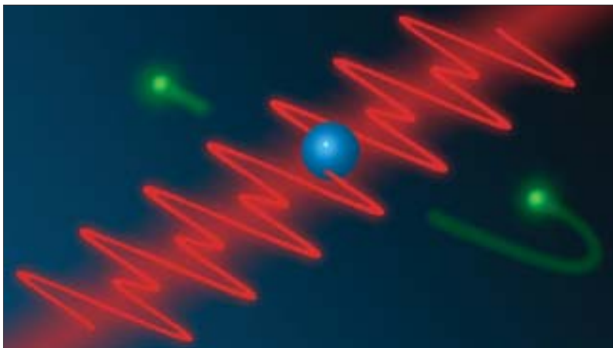
Durch Tunnelionisation von Atomen (blau) in einem Laserfeld (rot) erzeugte Elektronenpaare (grün) sind durch die Lichtoszillationen auf einer Attosekunden Zeitskala zueinander synchronisiert.
