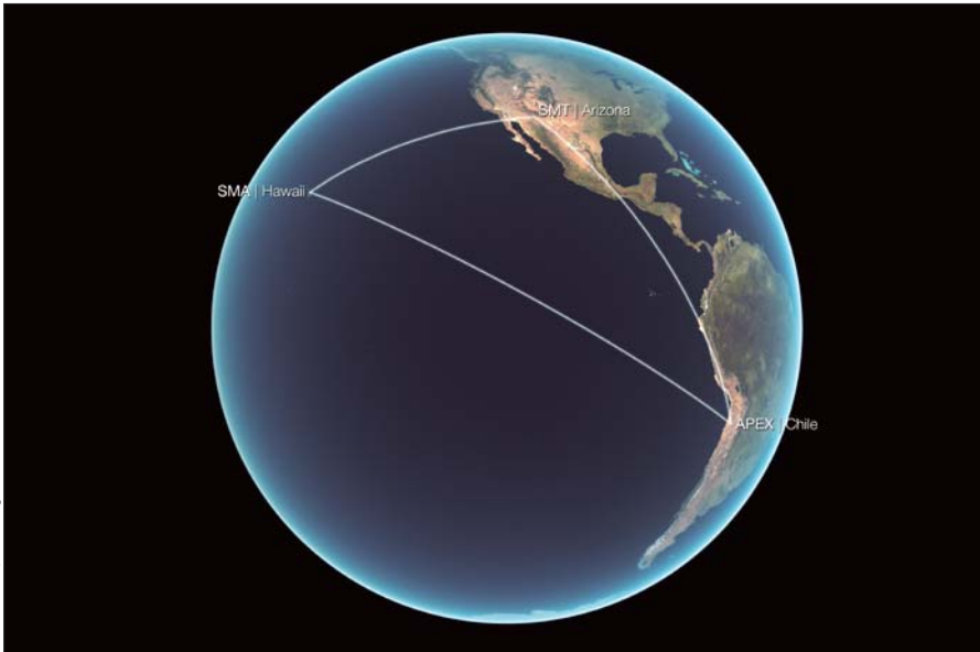
Positionen der drei an dem 1,3-mm-VLBI-Experiment beteiligten Radioteleskope: Die Basislinie zwischen Chile (APEX) und Hawaii (SMA) beträgt 9447 km, zwischen Chile und Arizona (SMT) 7174 km und zwischen Arizona und Hawaii 4627 km.
