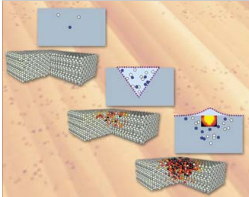
Niedrig geladene Ionen (links oben) führen nur zu kleinen Defekten in der Oberfläche, höher geladene Ionen stören das Material so stark, daß Teile weggeätzt werden können (Mitte) und hochgeladene Ionen tragen so viel Energie, daß das Material lokal aufgeschmolzen wird und Hügel ausbildet (unten rechts).
