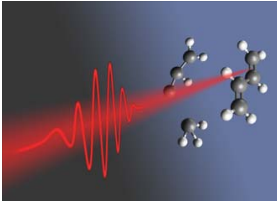
Ein kurzer Laserpuls trifft auf ein Molekül (hier: Butadien), das in zwei Bruchstücke zerfällt
