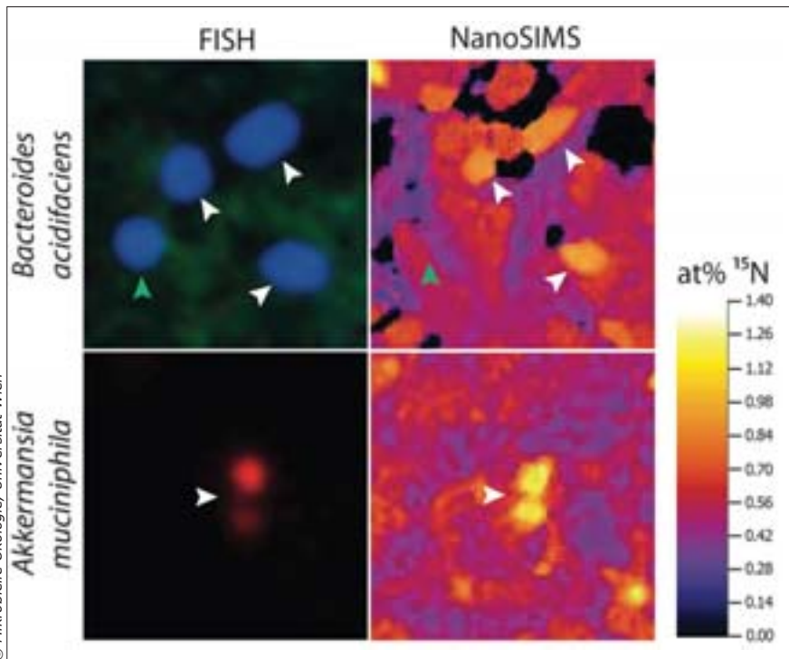
Korrespondierende FISH- (links) und NanoSIMS- (rechts) Analysen von Darmmikroorganismen. Bacteroides bzw. Akkermansia -Zellen wurden mit Hilfe von Gensonden und FISH spezifisch angefärbt. Der Gehalt derselben Zellen am stabilen Isotop ^{15}\text{N} wurde mittels NanoSIMS analysiert. Je höher der ^{15}\text{N} -Gehalt einer Zelle, desto mehr Darmschleim wurde von ihr aufgenommen. Weiße Pfeile zeigen auf Zellen, die Schleim aufgenommen haben. Die mit einem grünen Pfeil markierte Bacteroides -Zelle hat sich nicht von Schleim ernährt.
