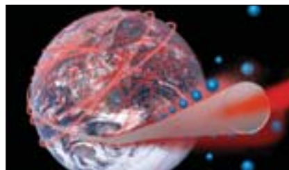
Datenhighways für Quanteninformation S 84
