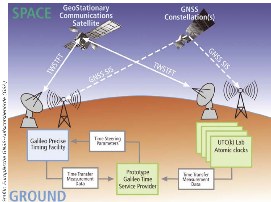
Darstellung des Galileo-Prinzips der Europäischen GNSS-Aufsichtsbehörde
