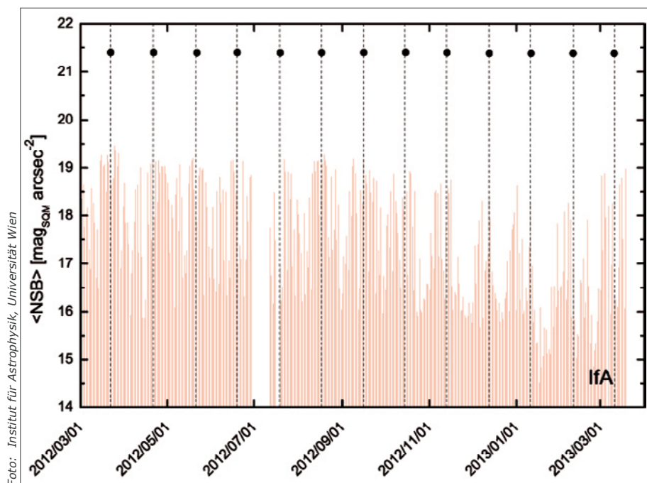
Klar ausgeprägte Monats-Periodizität in der mittleren Nachthimmelshelligkeit über dem Mitterschöpf, dem höchsten Berg des Wiener Waldes. Die schwarzen Kreise markieren die Neumond-Zeitpunkte. Hohe rote Balken stehen für dunkle Nächte.
