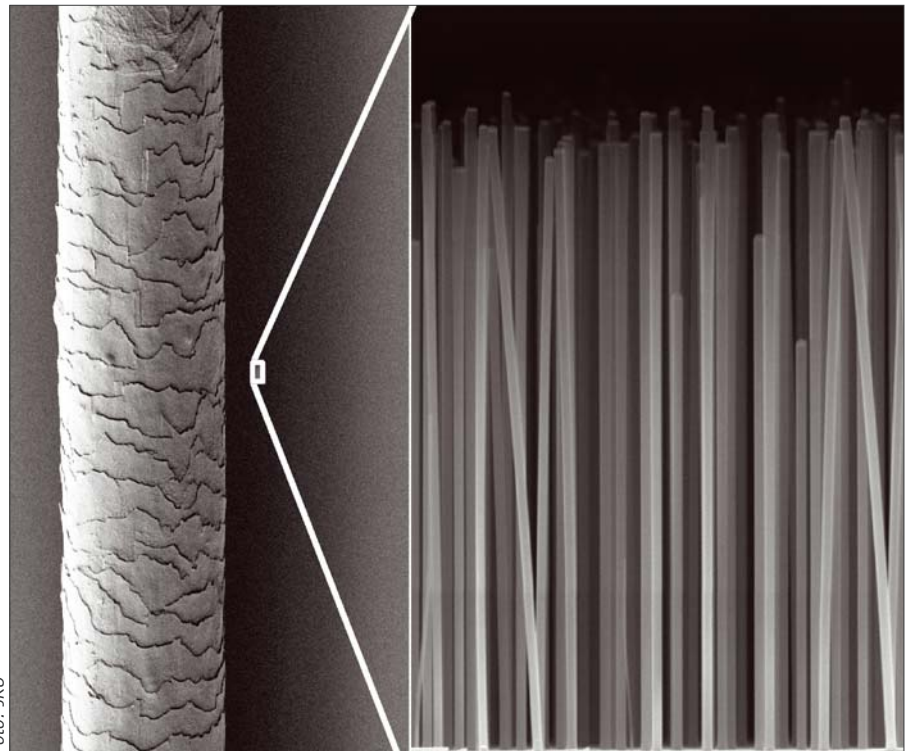
Elektronenmikroskopaufnahme eines menschlichen Haars im Vergleich mit der untersuchten Galliumphosphid-Nanostruktur welche etwa 1000mal dünner ist.
