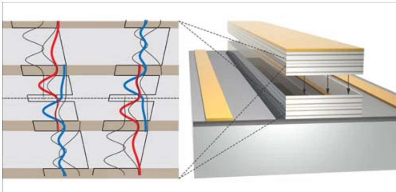
Zwei Laser werden zu einem verbunden. Links ist das symmetrische Schichtsystem dargestellt.
