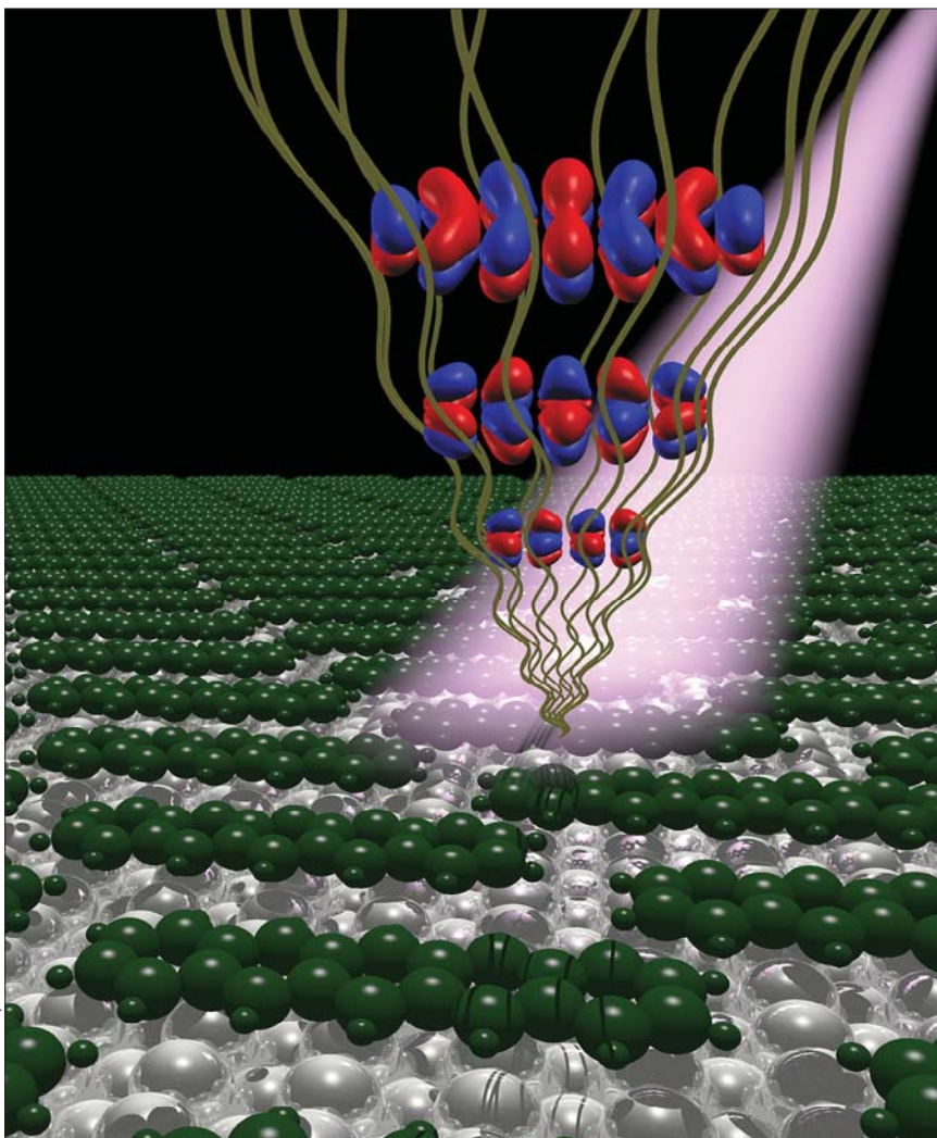
Ultraviolette Photonen schießen Elektronen aus einer Molekülschicht (grün) heraus, die auf einer Silberoberfläche adsorbiert ist. Die Messung der Energie- und Winkelverteilung der emittierten Elektronen liefert nach Anwendung eines iterativen mathematischen Verfahrens, die Elektronenorbitale des Moleküls (rot / blau).
