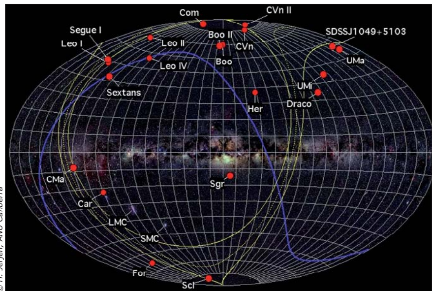
Die »Disk of Satellites« um die Milchstraße
