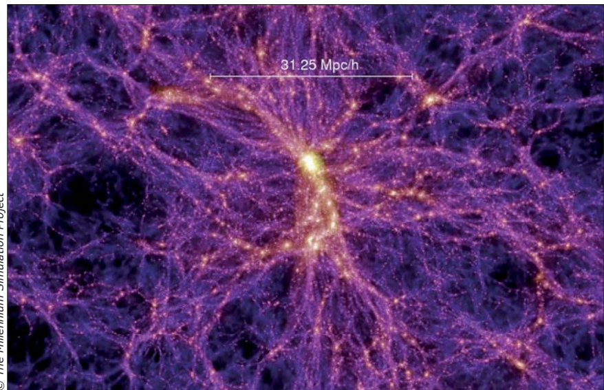
Das filamentförmige Cosmic Web in der Millenium-Dunkle-Materie-Simulation
