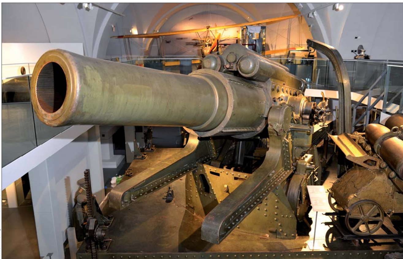
Das größte im Heeresgeschichtlichen Museum verwahrte Geschütz: eine 38 cm Haubitze.
