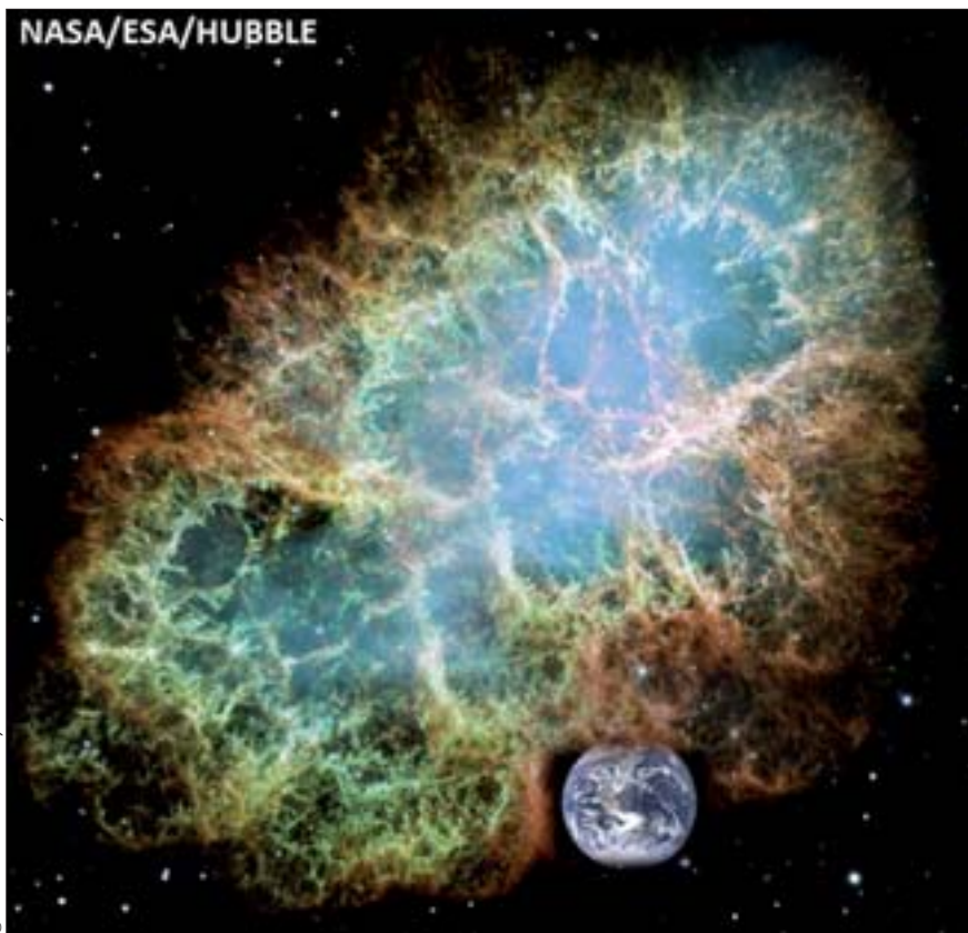
Die Fotocollage illustriert, wie kosmischer Staub aus Supernova-Explosionen auf die Erde gelangt ist. Der Krebsnebel ist ein Supernova-Überrest aus dem Jahr 1054 A.D. in 6300 Lichtjahren Entfernung, aufgenommen mit dem Hubble Space Telescope. Die Erde eine Aufnahme der Apollo 17 Crew. Die Originalbilder sind NASA und ESA-Aufnahmen.
