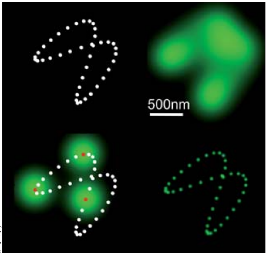
Die Grundidee: Wenn viele einzelne Punkte gleichzeitig leuchten (oben) dann ist bloß eine diffuse Wolke zu erkennen (oben rechts). Blitzen die einzelnen Punkte aber nacheinander auf (unten), dann kann man jeweils den Mittelpunkt berechnen und alle Punkte sauber abbilden (unten rechts).
