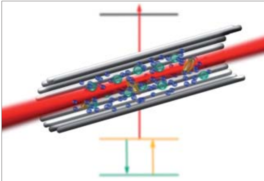
Schematische Darstellung der Ionenfalle, in der die kalten geladenen Moleküle mit Hilfe von Lasern untersucht werden.
