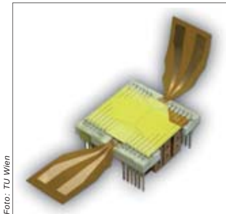
Atomchip zum Kühlen und Manipulieren der ultrakalten Atomwolken
