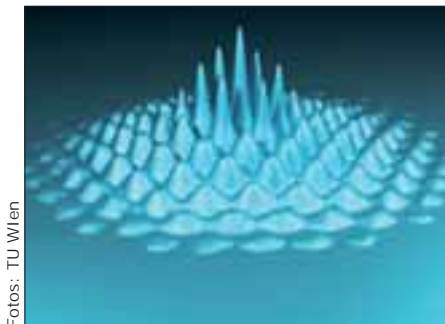
Ein Bose-Einstein-Kondensat schlägt Wellen
