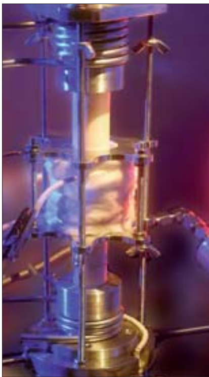
Beheizter Versuchsreaktor
