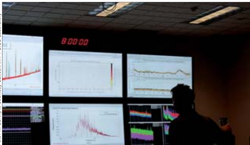
Foto: K. Burtnyk, Courtesy Caltech/MIT / LIGO Laboratory
