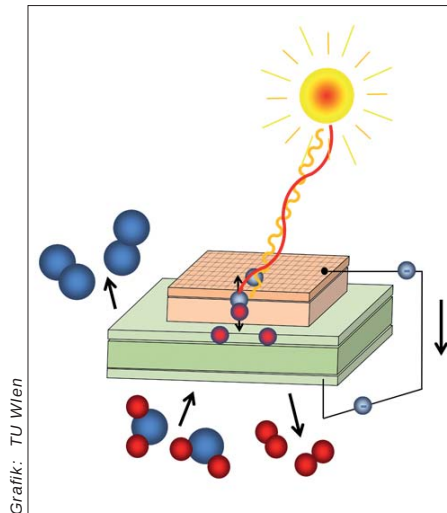
Photochemische Zelle: Licht erzeugt freie Ladungsträger, Sauerstoff (blau) wird durch die Membran gepumpt.
